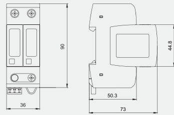
外形尺寸图
