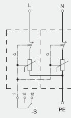
电气原理图
