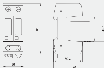
外形尺寸图
