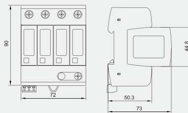
外形尺寸图
