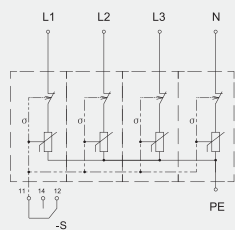
电气原理图
